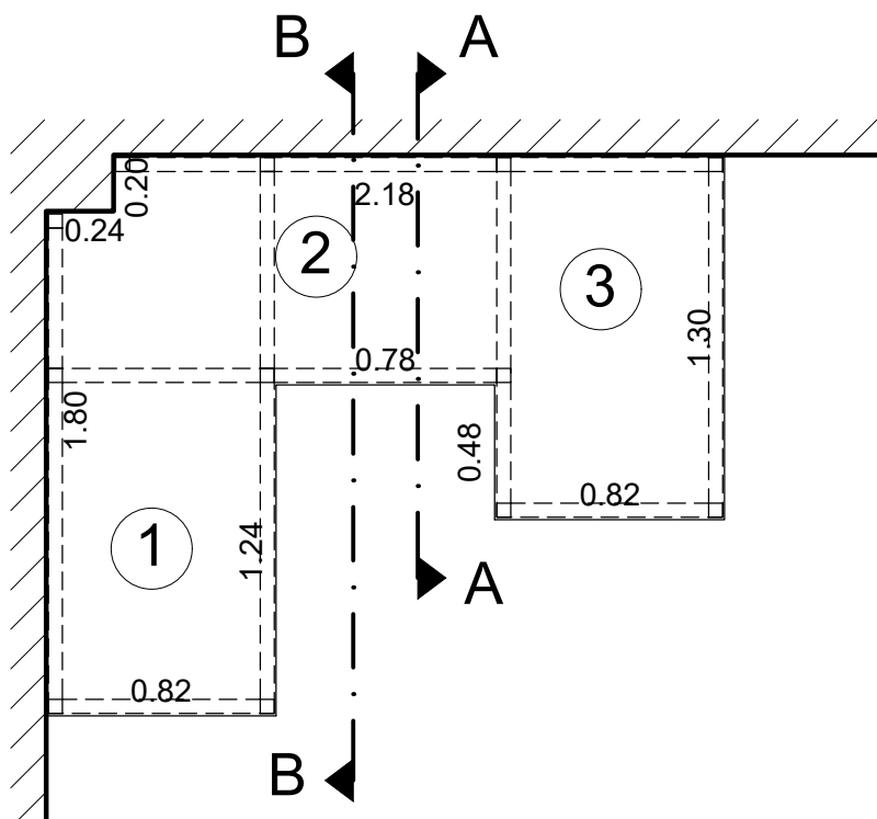
κάτοψη γραφείου
